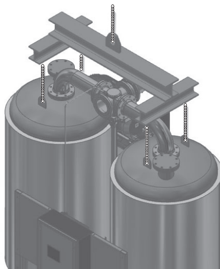
Transport dźwigiem
